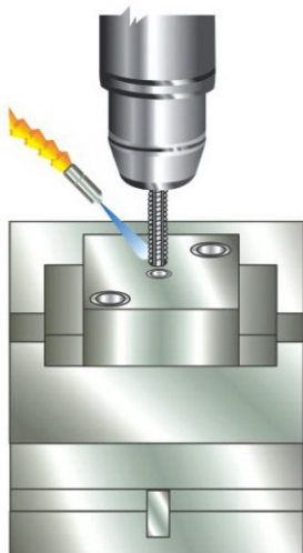
TAPPING
